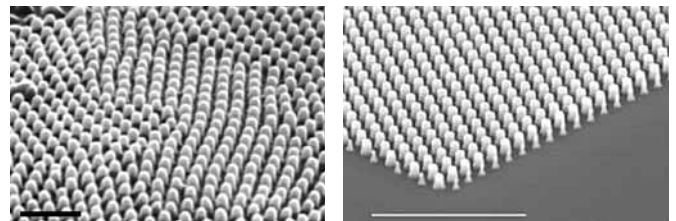
Abb. 10 links: Rasterelektronenmikroskopische Aufnahme der Oberfläche des Mottenauges. Länge des Skalierungsbalkens 1 \mu\text{m} [10].
