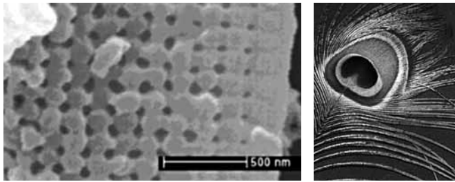
Abb. 7 links: Melaninzylinder mit 150 nm Abstand aus dem grünen Bereich einer Pfauenfeder.
