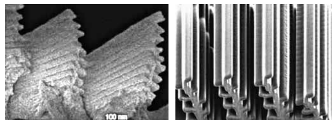
Abb. 11 links: Farbgebende Strukturen im Morpho-Schmetterling. Länge des Skalierungsbalkens 100 \text{ nm} [11].
